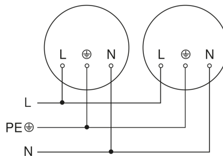
Schema elettrico
